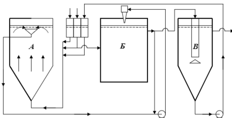
Схема нитри-денитрификатора
